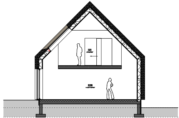
DWARSDOORSNEDE
