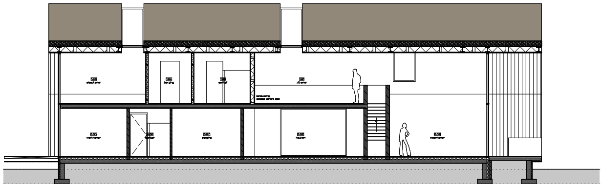
LANGSDOORSNEDE
